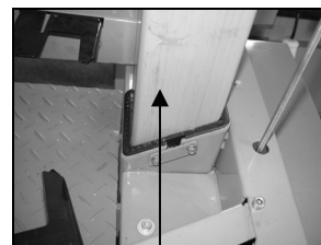
A hasító oszlop kenése
